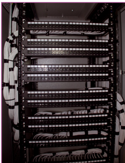
AfB. 2A: Patchkast...
